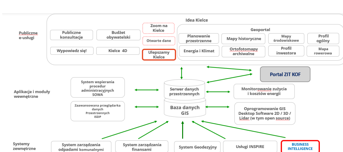
Rysunek 3 Schemat podstawowych modułów oraz funkcjonowania Miejskiego Systemu Informacji Przestrzennej.
